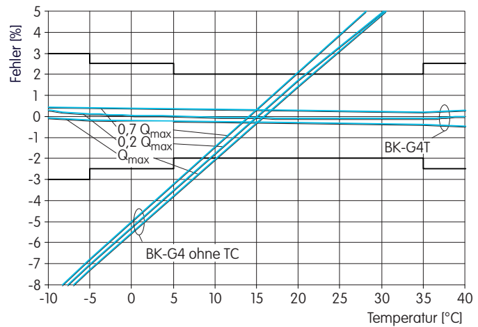
Messfehlerkurve BK-G4T im Umwertungsbereich mit Eichfehlergrenzen nach MID und DIN EN 1359:2007, Anhang B
