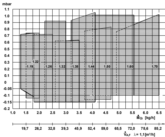
Abb. 50: Arbeitsfeld der Raketenbrenner® RE 1H / HK / HG
