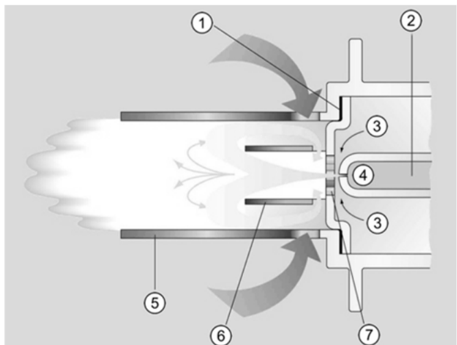
Abb. 52: Verbrennungsablauf Raketenbrenner®
