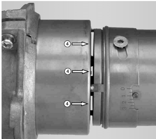
Abb. 9: Rezirkulationsschlitze ④
