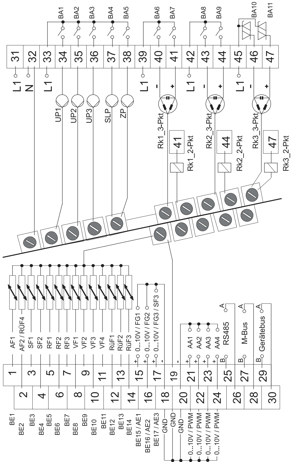
Bild 5: Elektrischer Anschluss des Heizungsreglers TROVIS 5578-1114
