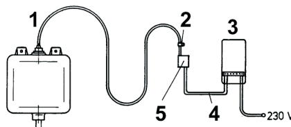
Bild 9: Schwarzer LAG-Behälter und Steuergerät nebeneinander montiert. Signalleitung lose, damit Sonde herausgenommen werden kann.
